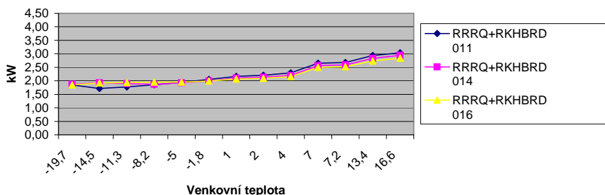
Porovnání účinností 011 + 014 + 016 při spádu 75/65°C
