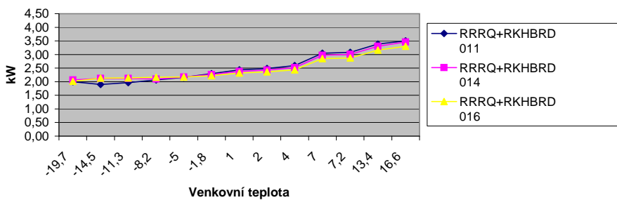
Porovnání účinností 011 + 014 + 016 při při spádu 65/55°C
