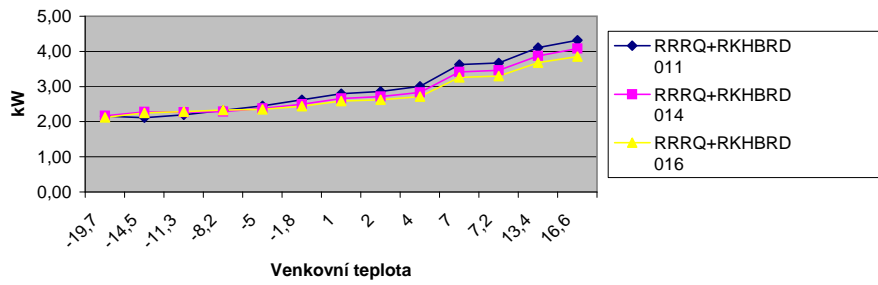
Porovnání účinností 011 + 014 + 016 při při spádu 45/40°C
