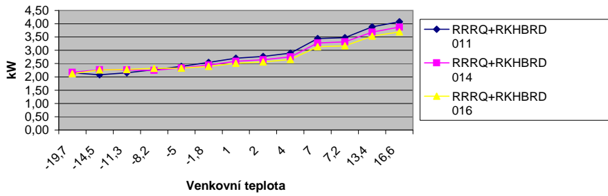
Porovnání účinností 011 + 014 + 016 při při spádu 55/45°C
