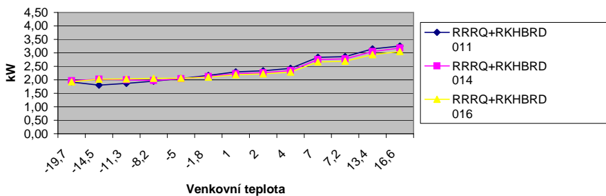
Porovnání účinností 011 + 014 + 016 při spádu 70/60°C
