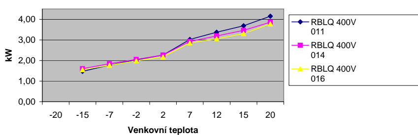
Porovnání účinností 011 + 014 + 016 pro vodu 50°C
