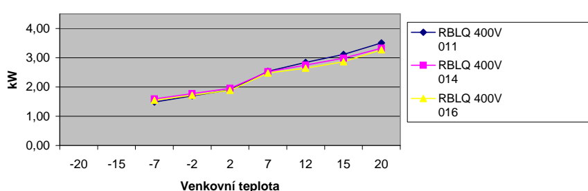
Porovnání účinností 011 + 014 + 016 pro vodu 55°C
