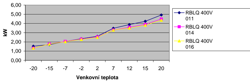
Porovnání účinností 011 + 014 + 016 pro vodu 45°C
