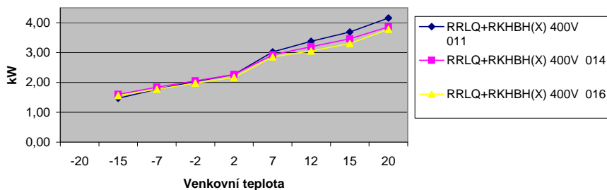
Porovnání účinností 011 + 014 + 016 pro vodu 55 °C
