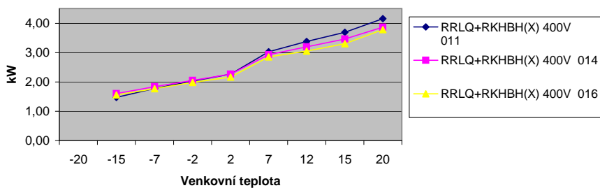
Porovnání účinností 011 + 014 + 016 pro vodu 50 °C
