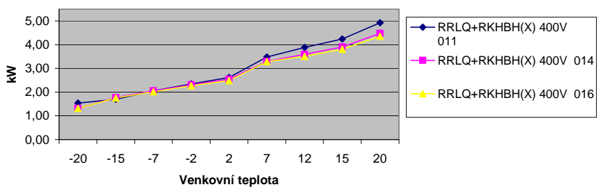
Porovnání účinností 011 + 014 + 016 pro vodu 45 °C
