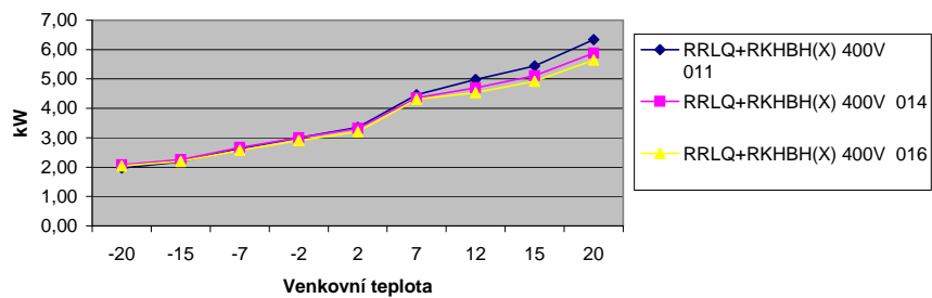
Porovnání účinností 011 + 014 + 016 pro vodu 35 °C
