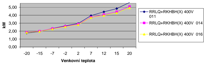
Porovnání účinností 011 + 014 + 016 pro vodu 40 °C
